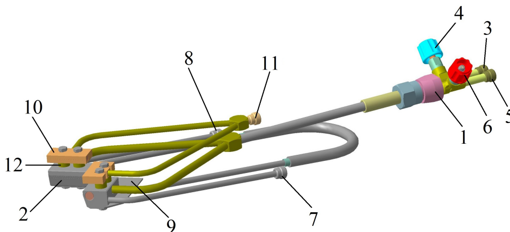
Рис.1. Горелка ГП-3з Угол
